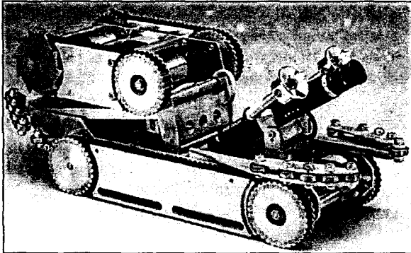
Илл. 33. Робот, который Гантенбринк использовал для изучения «шахт» Великой пирамиды. В честь таинственного египетского божества он назван Упуат
