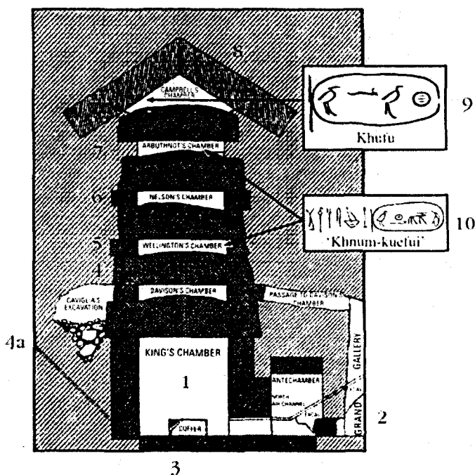
Рис. 8. Помещения в конструкции Великой пирамиды 1. «Царская палата». 2. Великая галерея. 3. «Гробница». 4. «Палата Дэвисона». 4а. Раскопки Кавигильи. 5. Палата Веллингтона. 6. Палата Нельсона. 7. Палата леди Арбатнот. 8. Палата Кемпбелла. 9. «Хуфу». 10. «Хнум куфуи»
